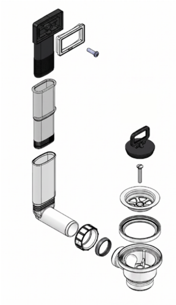
Piletta di scarico in polipropilene a una via con troppo pieno e scarico filettato da 1"1/2, completa di tappo.
